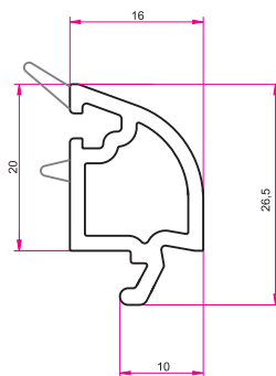
Çift Cam Çıtası Double Glazing Bead Штапик с уплотнителем (серого цвета) для одинарного стеклопакета
