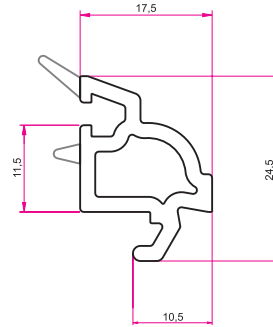
Çift Cam Çıtası Double Glazing Bead Штапик с уплотнителем (серого цвета) для одинарного стеклопакета
